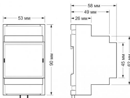
Габаритные размеры SH-CHO4.3IS1
