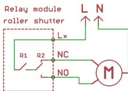
Пример схемы подключения SH-CHO4.3IS1
